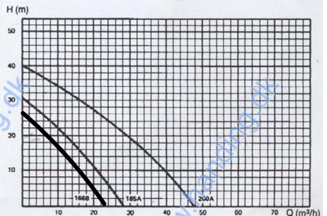
Fig. 2. Kapacitetsdiagram.
