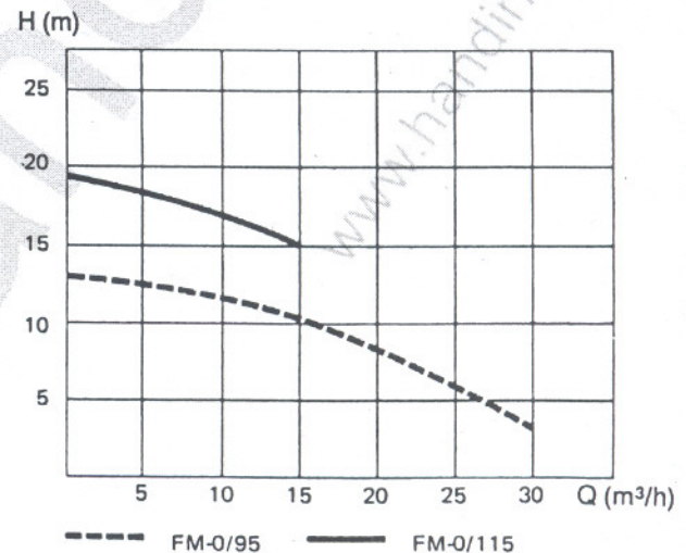
Fig. 2. Kapacitetsdiagram.
